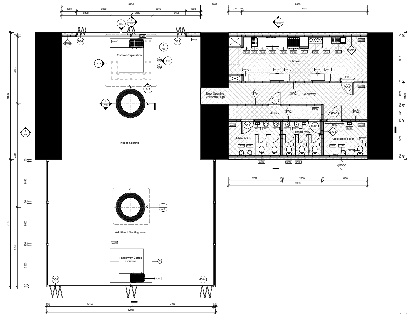
1 Floor Plan 1 : 50
