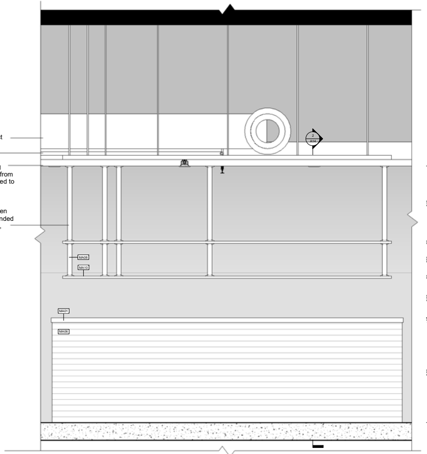
1 Elevation 1 1 : 10
