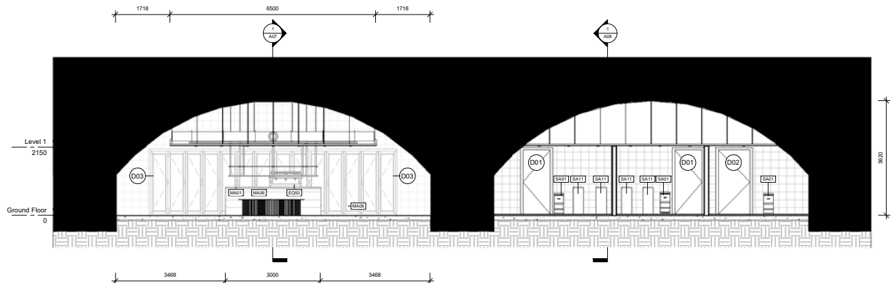
1 Section 1 1 : 50
