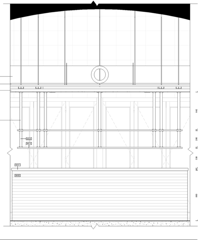
① Elevation 2 1 : 10
